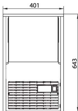
Vue frontale
